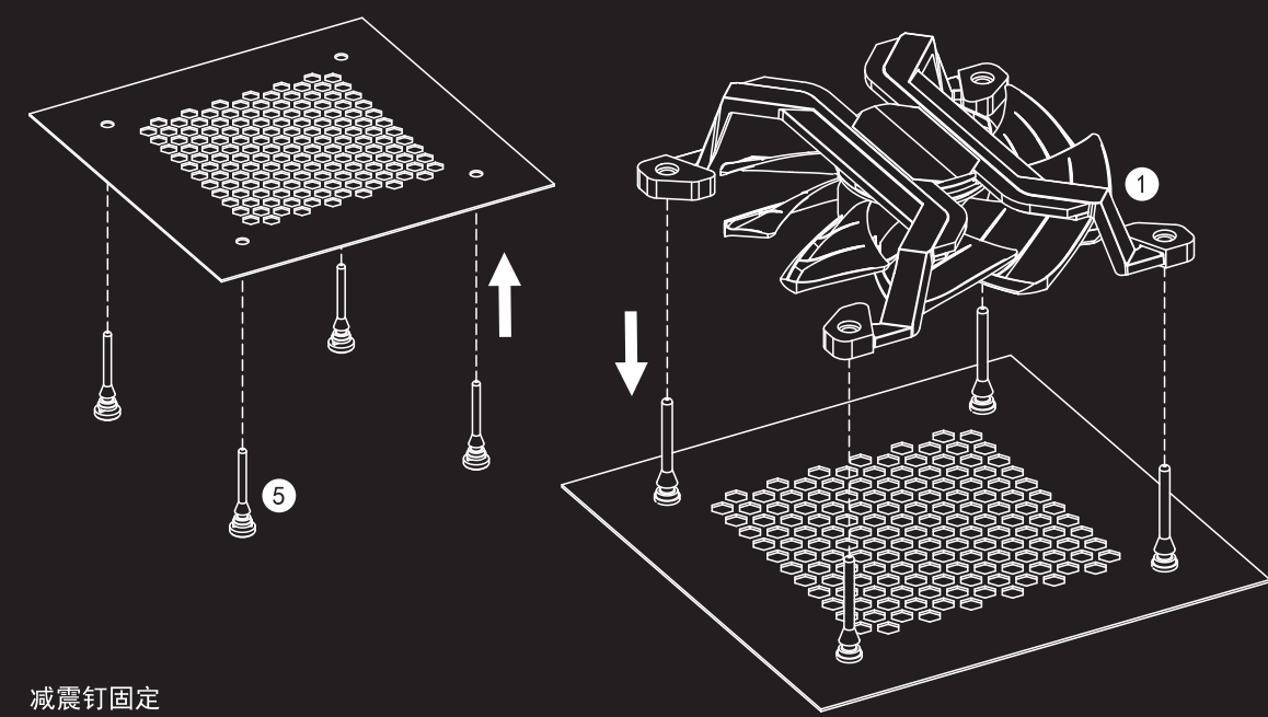
减震钉固定
